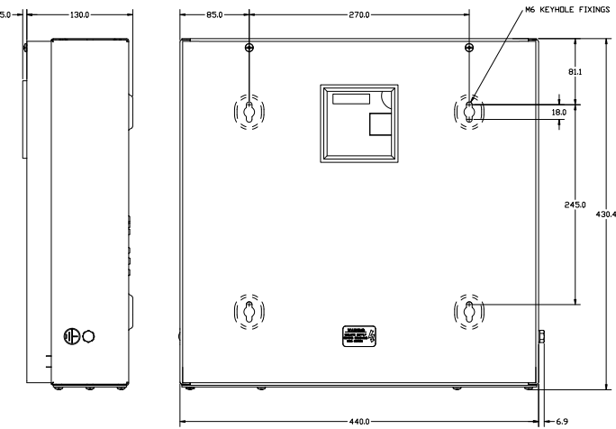
EBMMPCD120
