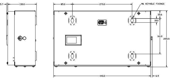
EBMMPCT250/EBMMPCT250M/EBMMPCT250MID
